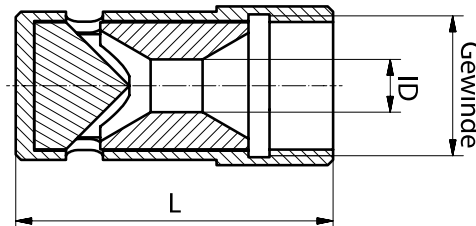
Strahlkopf mit 2 Auslassöffnungen mit G 3/4" Innengewinde
