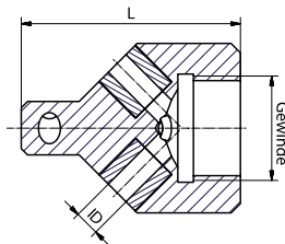
Strahlkopf mit 4 Auslassöffnungen und 1" Innengewinde
