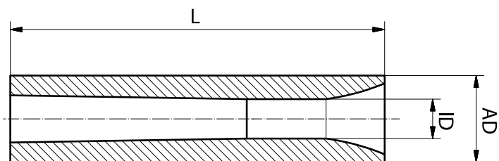
Einsatz Laval kurz
