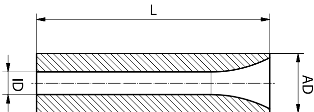
Einsatz mit großem Konus
